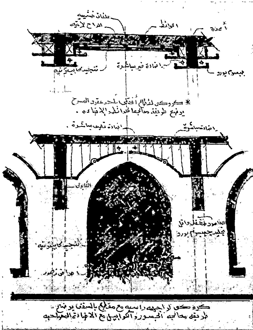
شكل رقم (10) استكش يوضح المعالجة الرأسية للفراغ بين الأعمدة وكذلك المعالجة الأفقية للسقف والتي شكلت فيما بينهما تجانسا جماليا ووظفيا.
